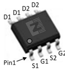
SOP8
